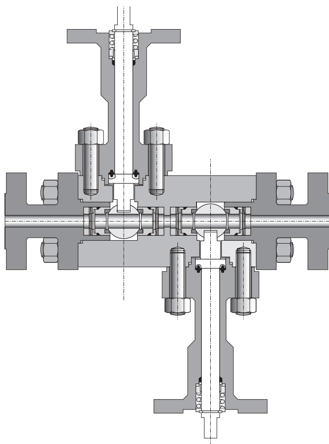
Sistema valvola a doppia sfera con drenaggio intermedio
